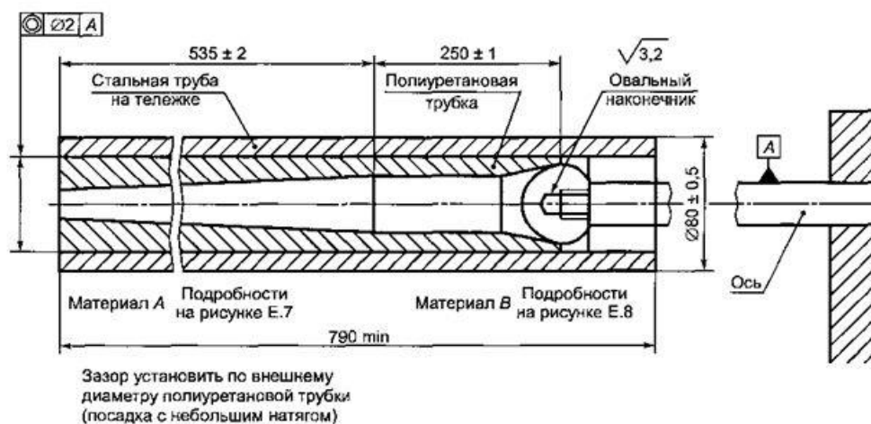
Рисунок Е.6 — Размеры стопорного устройства
