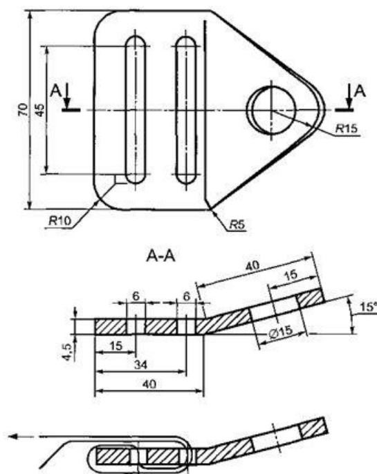
Рисунок П.2 — Стандартная пластина для крепления
