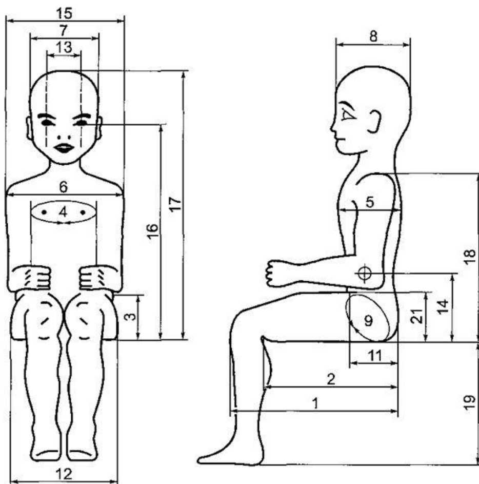
Рисунок И 1 — Основные размеры манекенов
