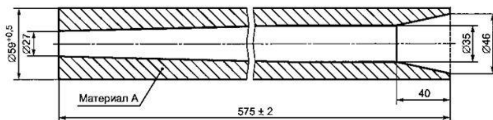
Рисунок Е.12 — Полиуретановая трубка
