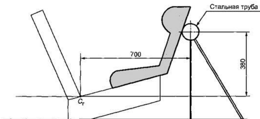
Рисунок Е.1 — Схема испытания детского удерживающего устройства, обращенного назад
