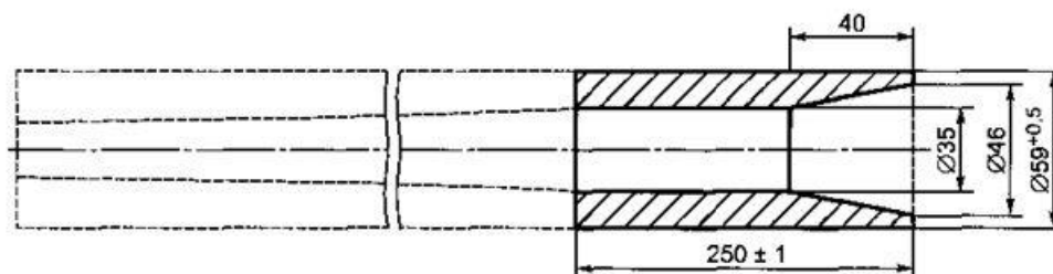
Рисунок Е.8 — Полиуретановая трубка из материала В
