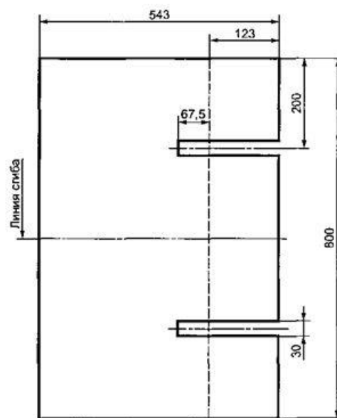
Алюминиевая пластина — толщиной (2,0 \pm 0,1) мм Угол изгиба — 15^\circ \pm 1^\circ
