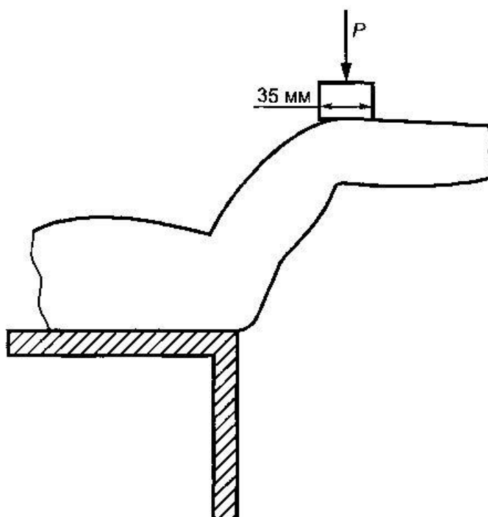
Рисунок И.12 — Калибровка жесткости сочленения ноги
