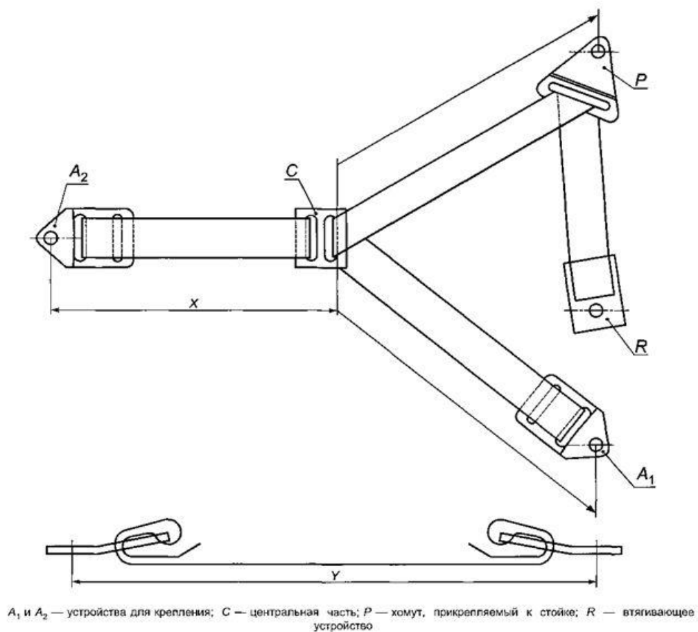
Рисунок П.1 — Конфигурация стандартного ремня безопасности
