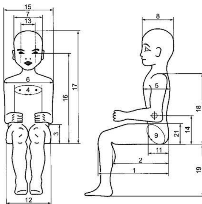
Рисунок И.13 — Основные размеры манекена 18-месячного ребенка
