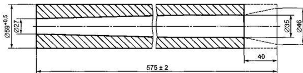
Рисунок Е.7 — Полиуретановая трубка из материала А
