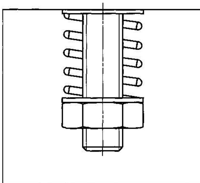
Рисунок И.8 — Регулирование поясничного троса
