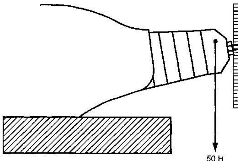
Рисунок И.2 — Регулирование троса шеи
