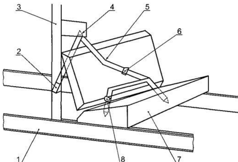
1 — испытательная тележка, 2 — стандартное затягивающее устройство, 3 — стойка В, 4 — хомут прикрепляемый к стойке, 5 — положение зажима, при наличии, 6 — датчик нагрузки № 2, 7 — подушка сиденья, предназначенная для испытания, 8 — датчик нагрузки № 1
