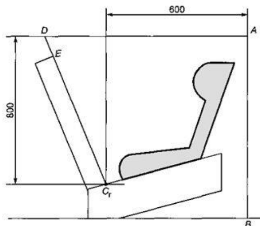
Рисунок 3 — Схема испытания детского удерживающего устройства, относящегося к группе 0, которое не упирается в приборную доску
