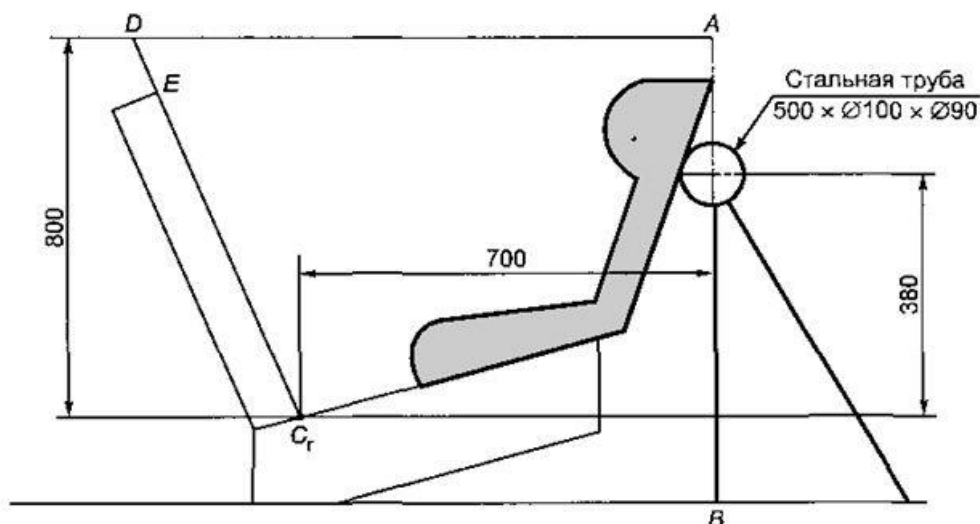
Рисунок 2 — Схема испытания детского удерживающего устройства, обращенного назад
