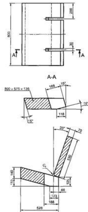
Рисунок Е.2 — Размеры сиденья и подушек сиденья
