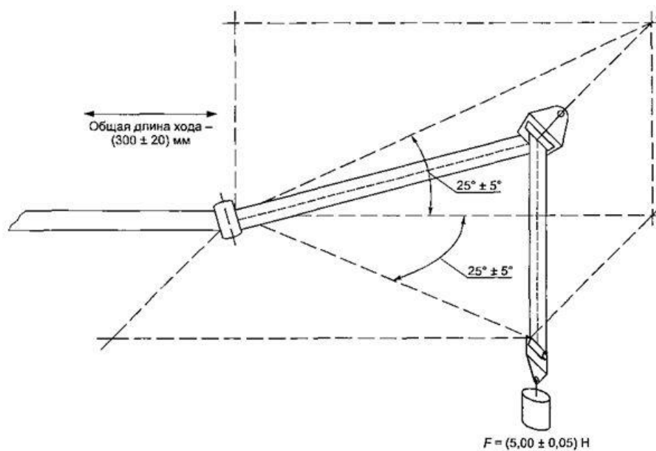
Рисунок Д.4 — Испытание с направляющим устройством
