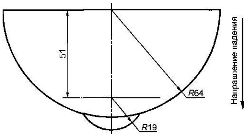
Рисунок Т.1 — Модель головы
