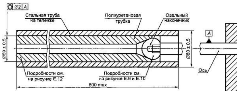
Рисунок Е.11 — Стопорное устройство в сборе
