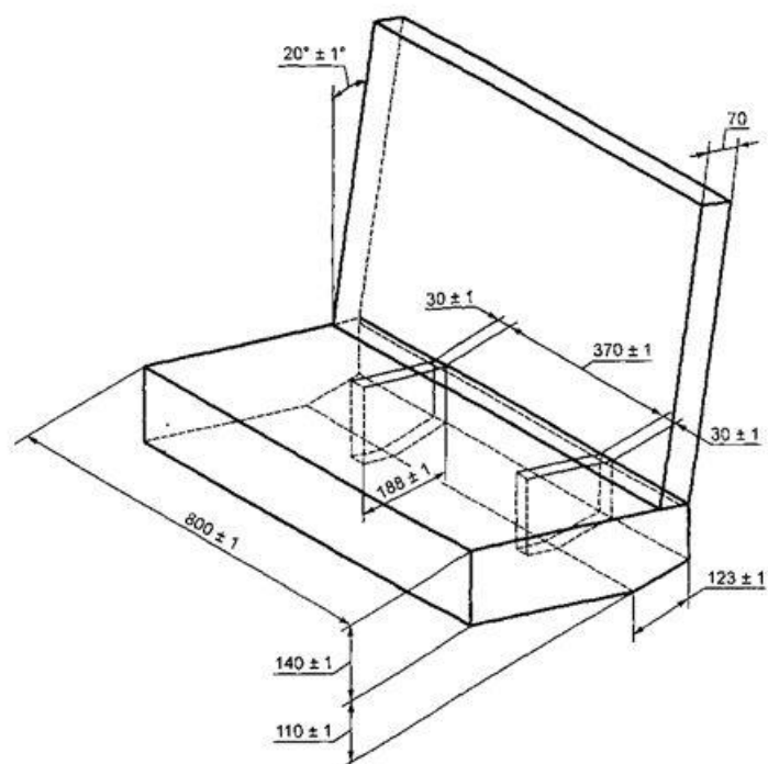
Рисунок Е 5 — Размеры сиденья (трехмерное изображение)
