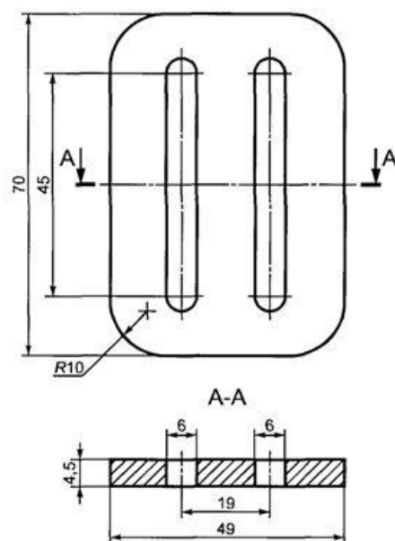
Рисунок П.3 — Центральная деталь стандартного ремня безопасности
