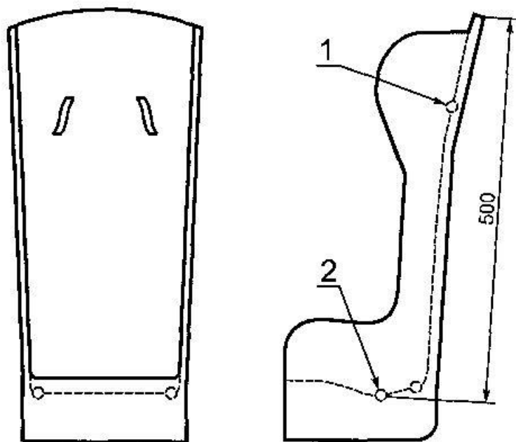
Рисунок Н.1 — Места крепления
