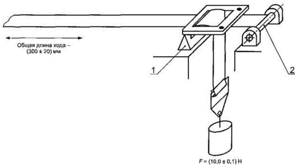
Рис. Д.1. Схема испытания А
