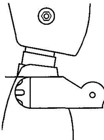
Рисунок И.6 — Регулирование плечевых сочленений
