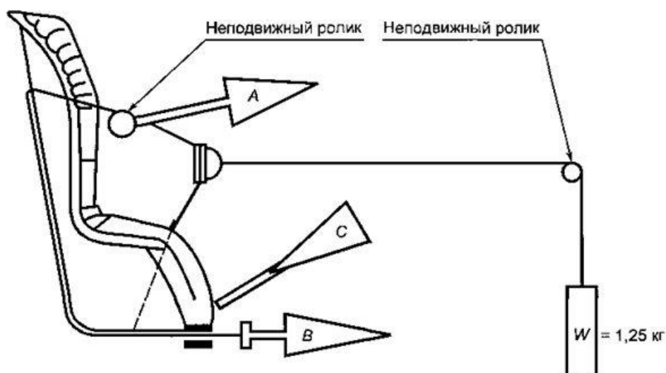
Рисунок X.1 — Схема испытательного устройства
