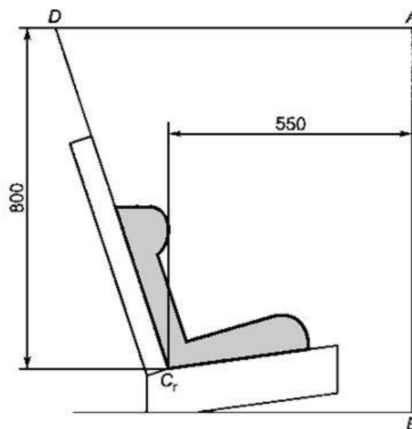
Рисунок 1 — Схема испытания детского удерживающего устройства, обращенного вперед
