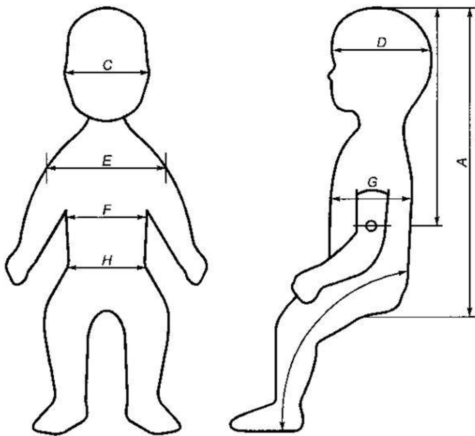
Рисунок И.10 — Манекен, моделирующий новорожденного
